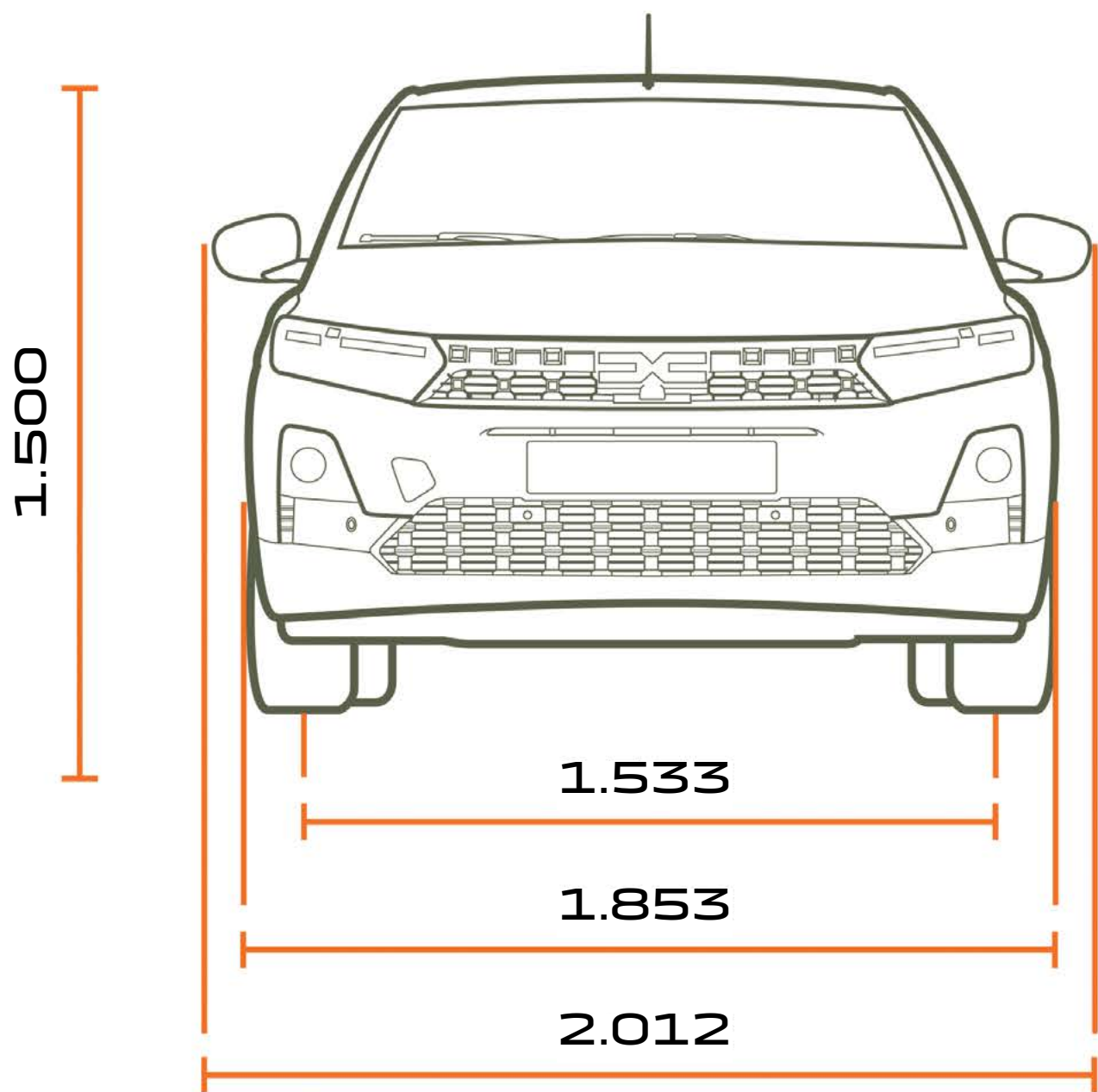
VEDERE FRONTALĂ
