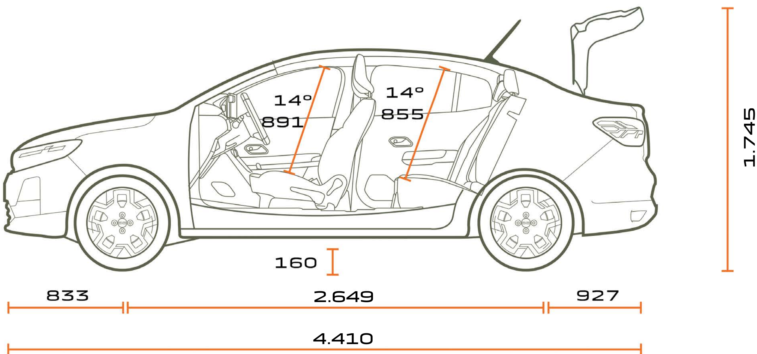
VEDERE LATERALĂ
