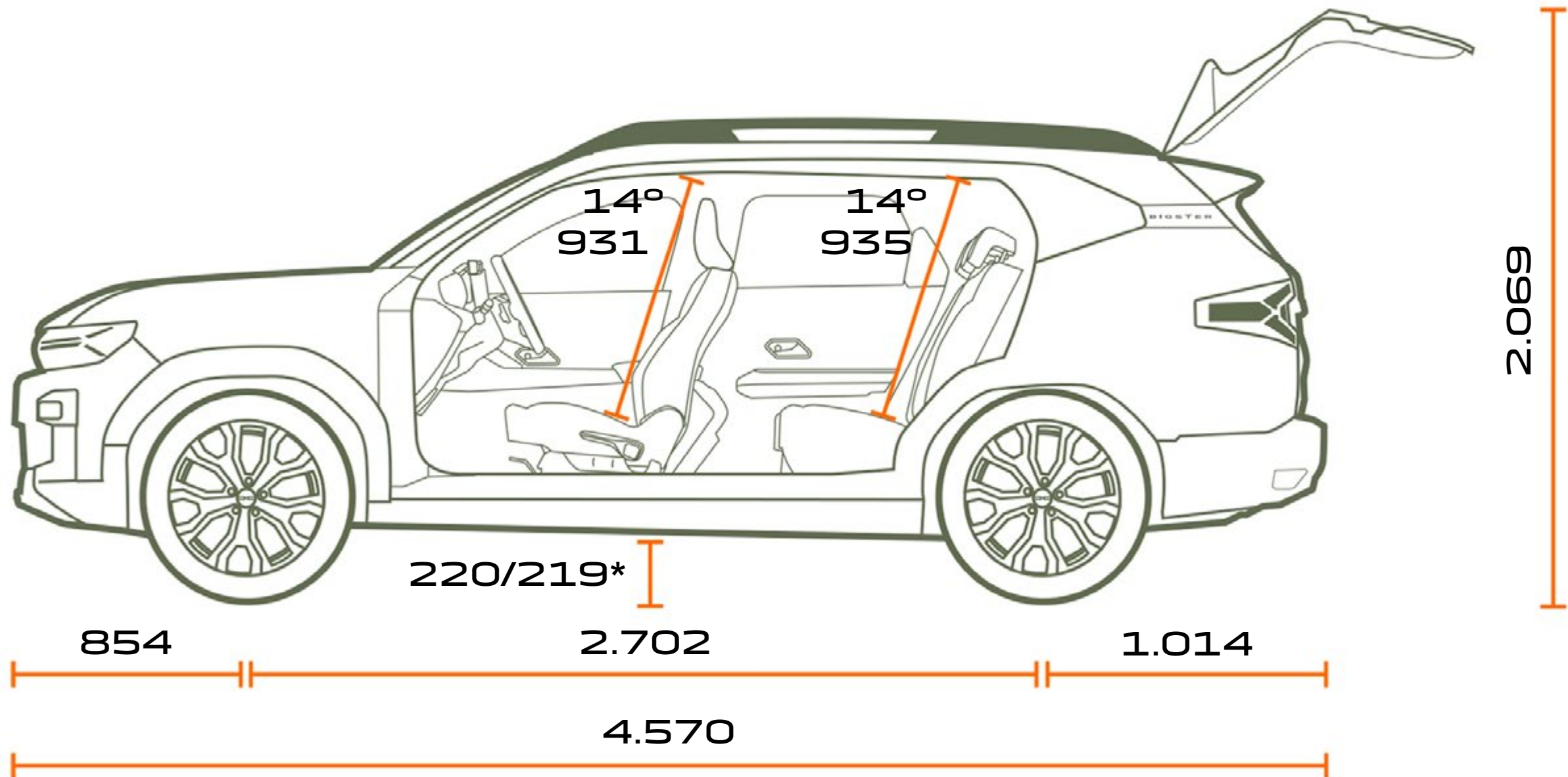
VEDERE LATERALĂ
