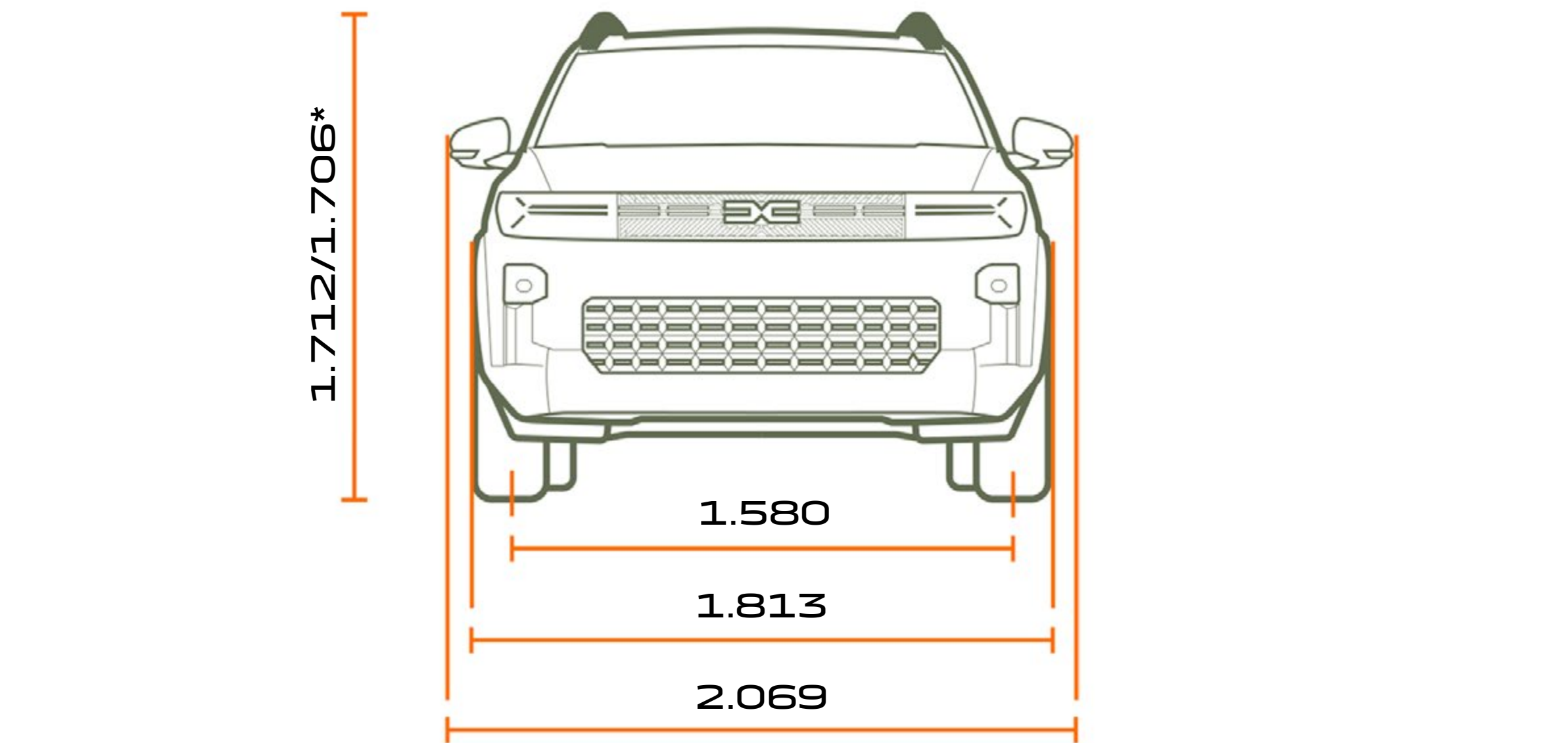
VEDERE FRONTALĂ
